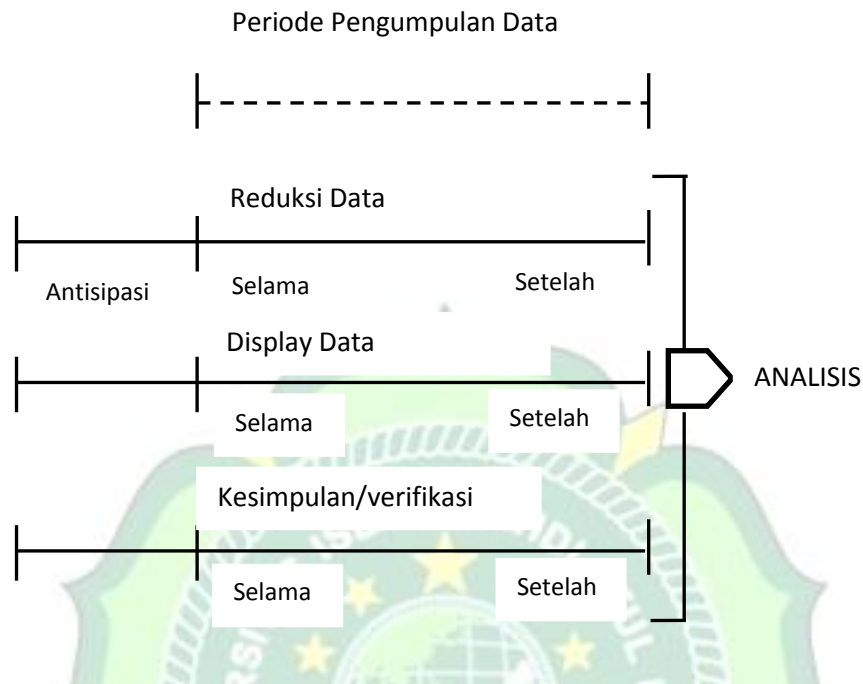
Gambar 3.2. Komponen dalam analisis data ( flow model )
